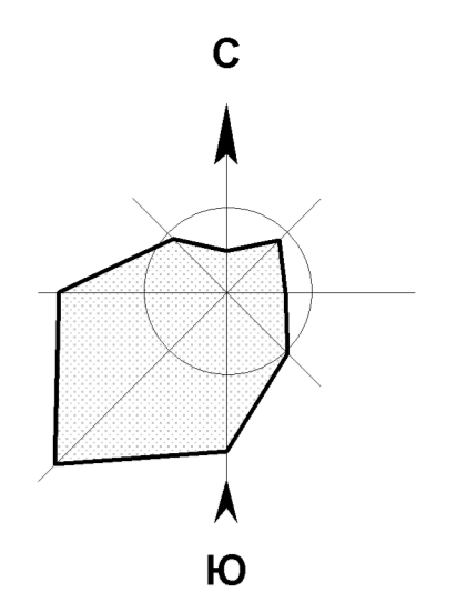
Среднегодовая роза ветров
